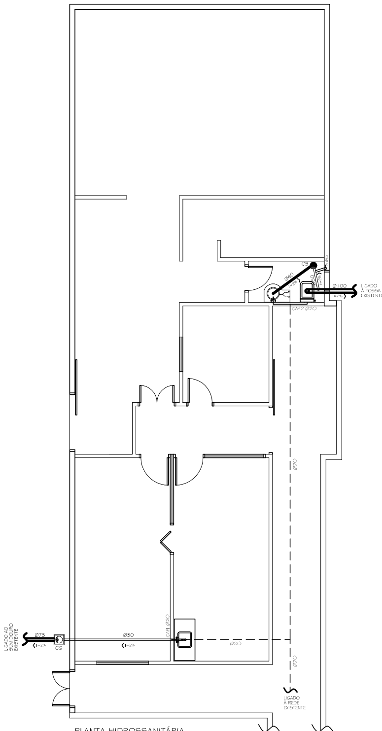
PLANTA HIDROSSANITÁRIA escala 1:50
